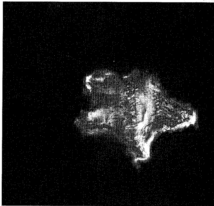
Fibra 32.9 corte transversal en extinción
